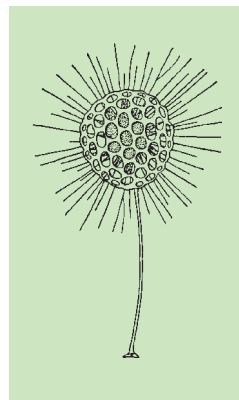
Рис. 6. Солнечник
