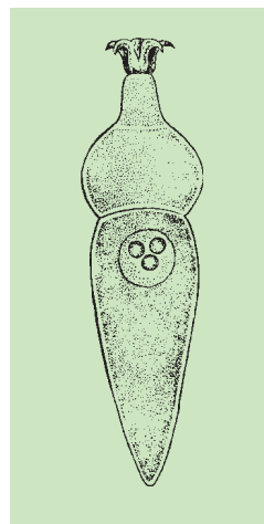
Рис. 7. Споровик грегарины
