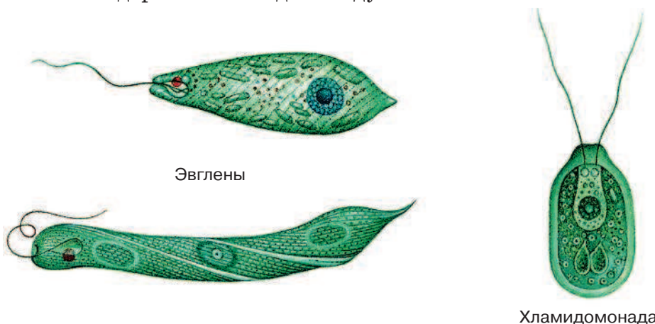
Рис. 8. Растительные жгутиконосцы
