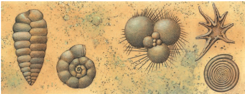
Рис. 4. Фораминиферы
